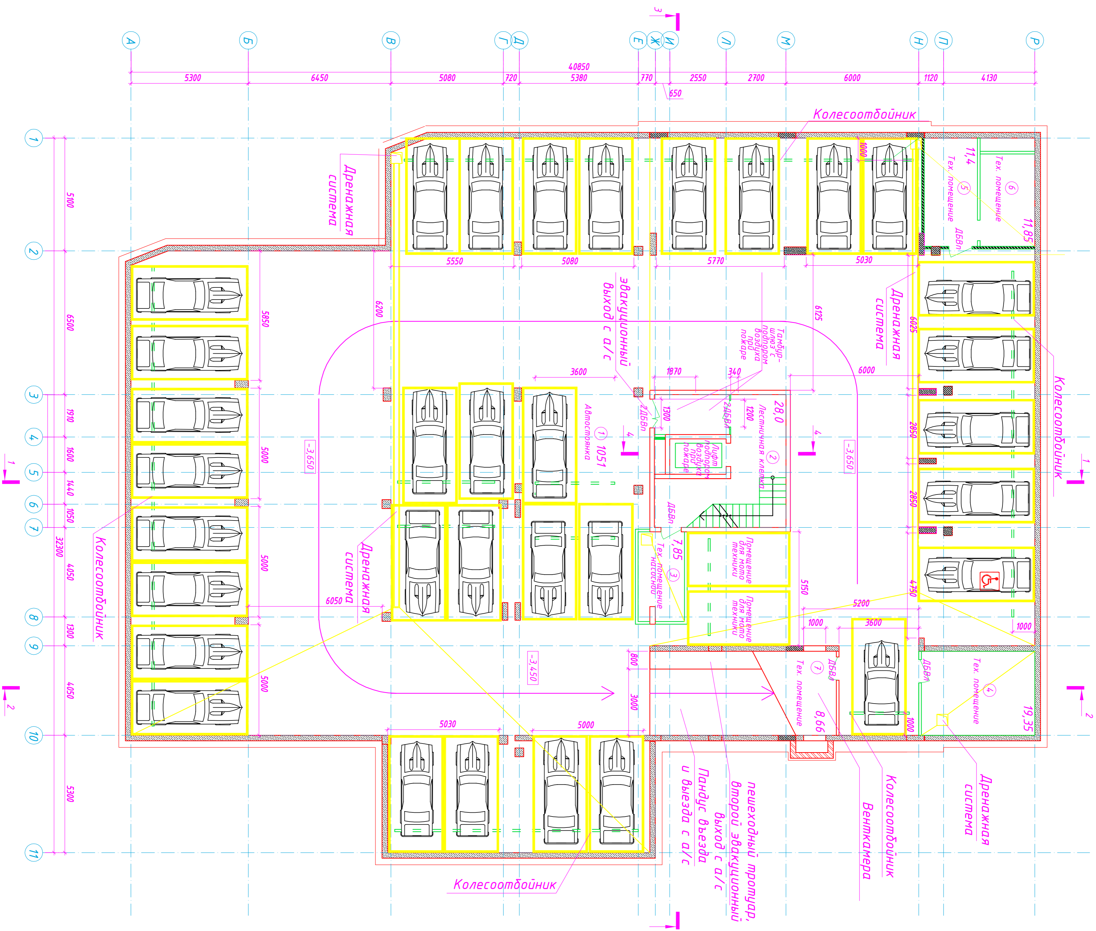
План автостоянки на отм. -3,650
